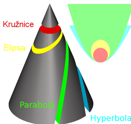
Obrázek 3: Kuželosečky
