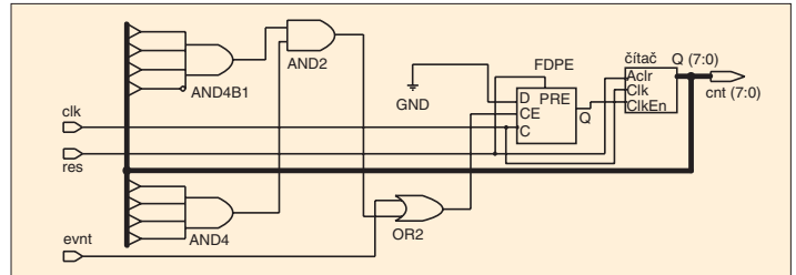
Obr. 3 Schéma RTL obvodu
